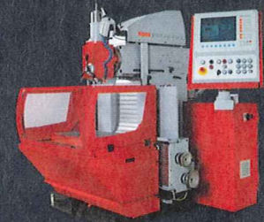
EMCOMAT FB 450-L Universal Werkzeugfräsmaschine mit EMCO-eigener Zyklensteuerung
