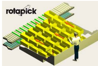
Hochleistungskommissioniersystem psb rotapick Funktionsprinzip psb rotapick Foto/Grafik: psb intralogistics GmbH)
